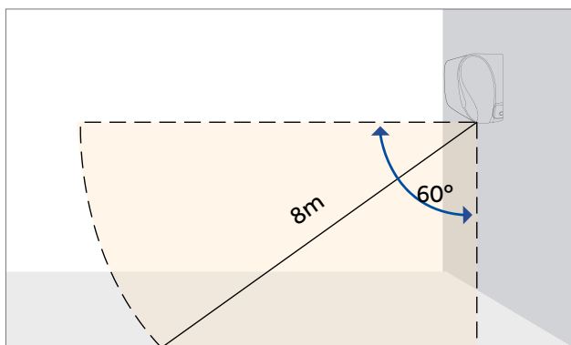
Obszar wykrywania w pionie
